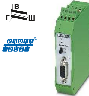
Активное терминирование шины для PROFIBUS и 2-проводных систем RS-485
