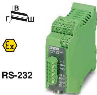
Последовательный расширитель
