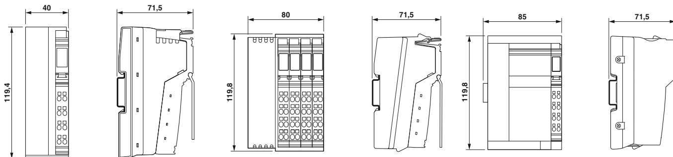
Корпус ВК
