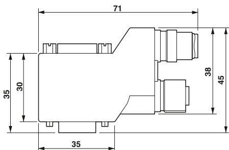
Размерный чертёж SUBCON-PLUS...90...M12, короткая модель 90°
