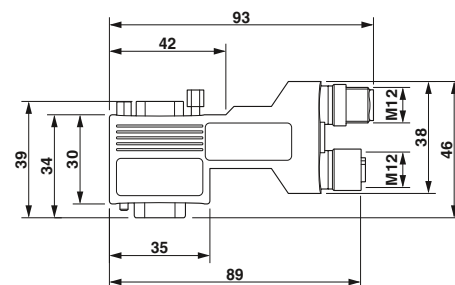
Размерный чертёж SUBCON-PLUS...90X...M12, длинная модель 90°
